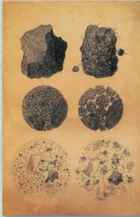
◀「岩石の風化」左列は新鮮な安山岩。右列は風化した安山岩。上段が肉眼、中段がルーペ、下段が偏光顕微鏡で見た図
