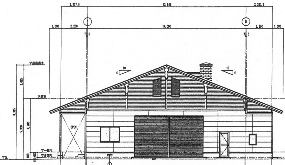
西立面図 1:100
