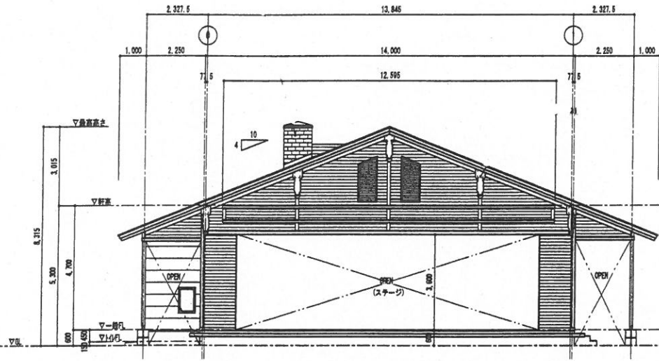
東立面図 1:100
