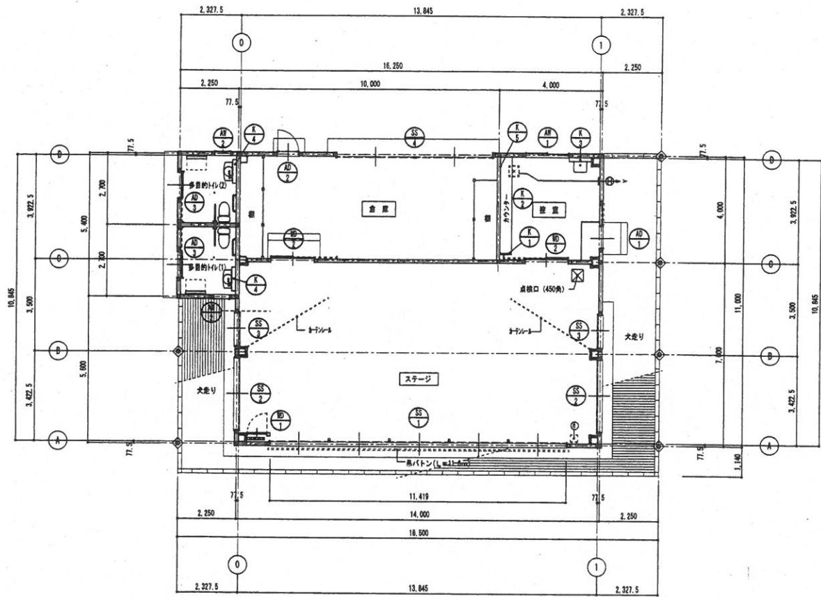
平 面 図 1 : 100
