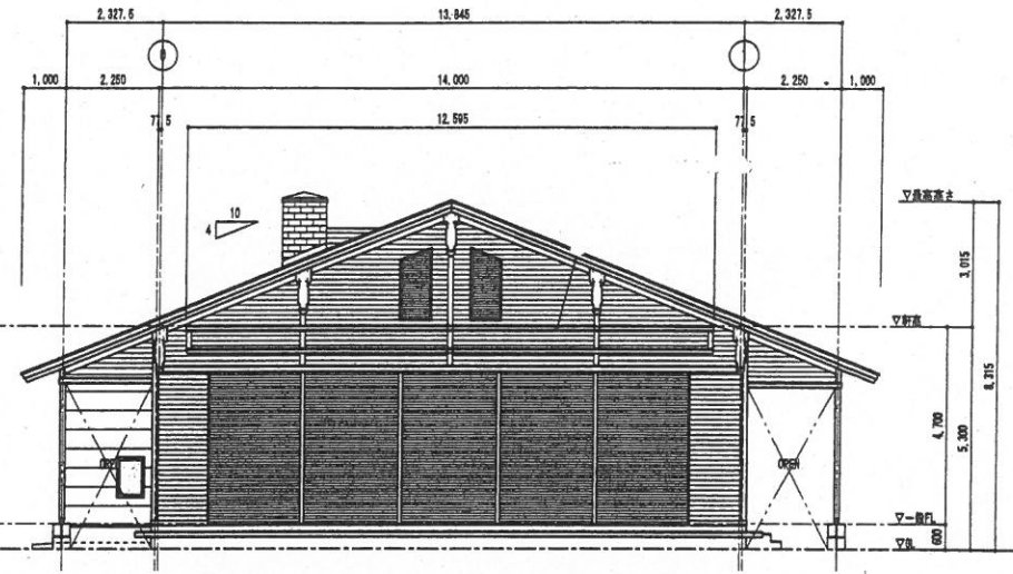
東立面図 1:100
