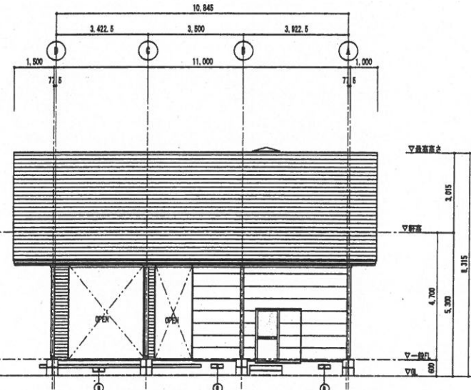
北立面図 1:100
