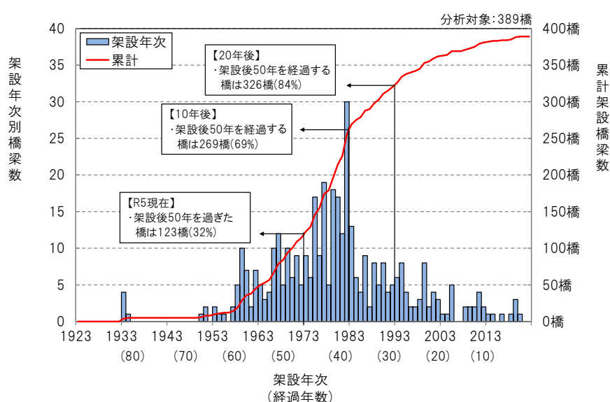
▲ 架設年次別橋梁数の分布
