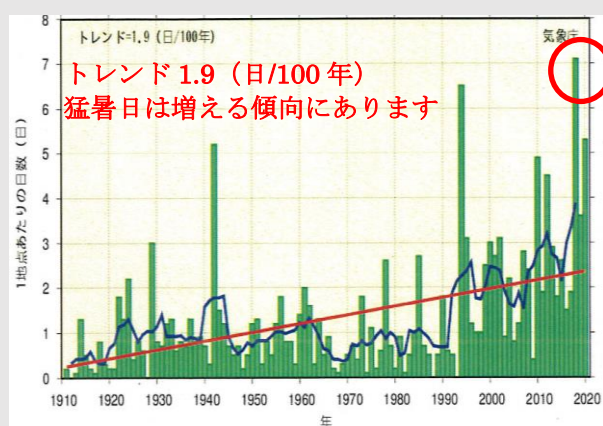
図 全国の日最高気温35℃以上(猛暑日)の年間日数の経年変化(1910～2020年)
