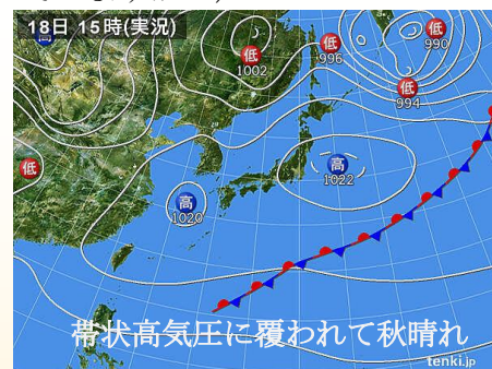
令和5年10月18日15時の地上天気図（盛岡の日照時間8.3時間）
