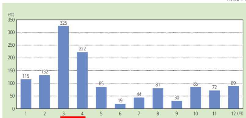
第1-1-18図 林野火災の月別出火件数
