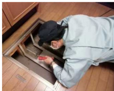
「土台・床組、基礎」調査の様子
