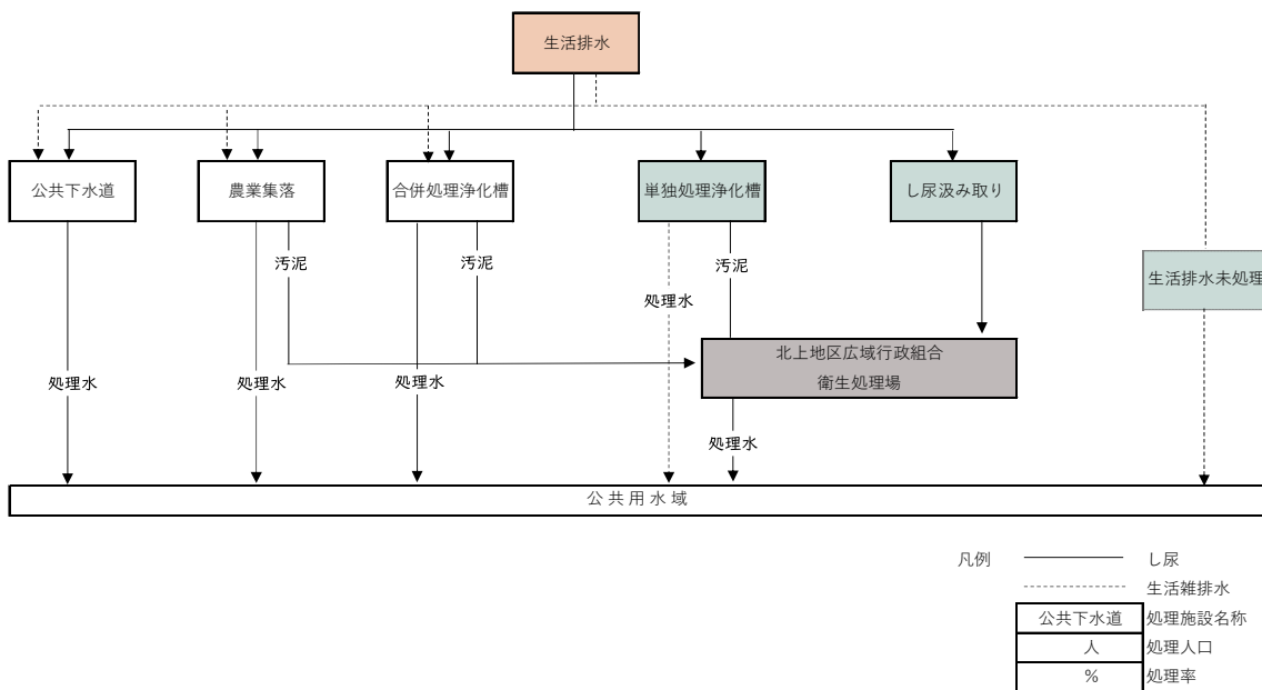
図 5-1 生活排水処理フロー
